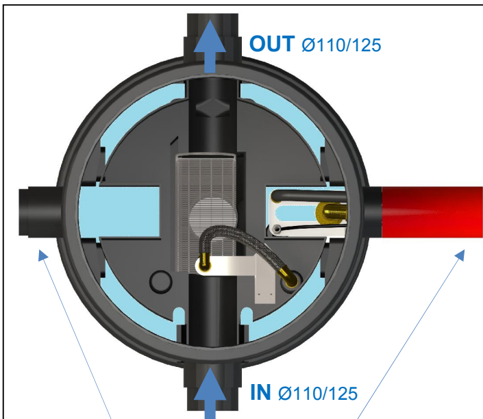
Aansluiting Mantelbuizen Connection casing tubes Anschluß Lehrrohren Ø110 mm
