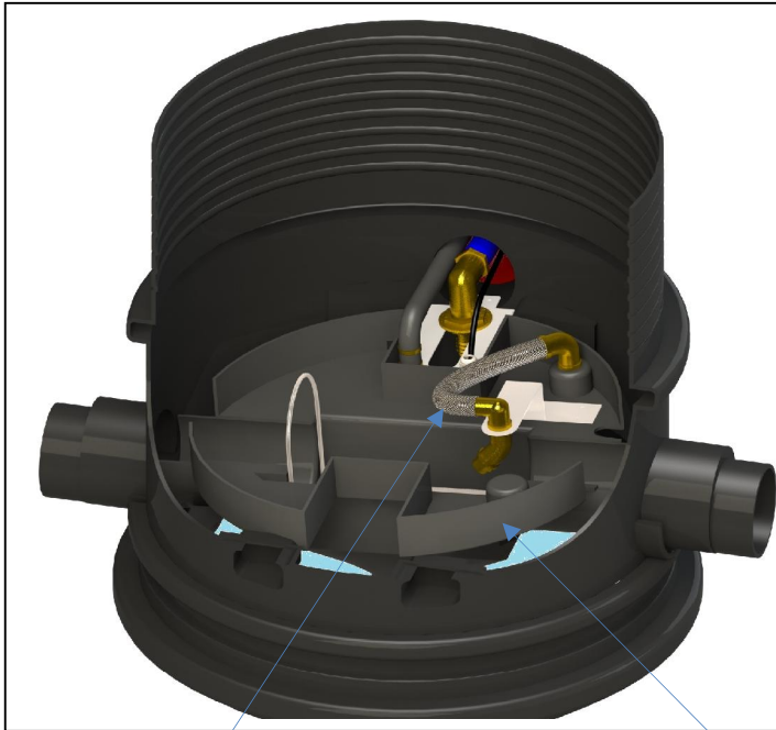
Filterreinigungsset Filtercleansingset Filterreinigungsset
