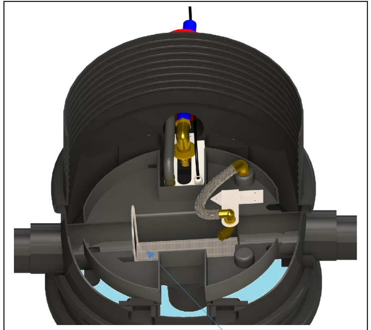
Kinderveilige filterschotel, uitneembaar Childsafe filterdish, removable Kindersichere Filterebene, ausnehmbar
